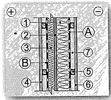
Рис. 3 Утепленная каркасная стена
