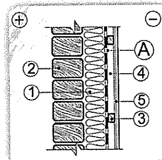
Рис. 4 Брусчатая стена с наружным утеплением
